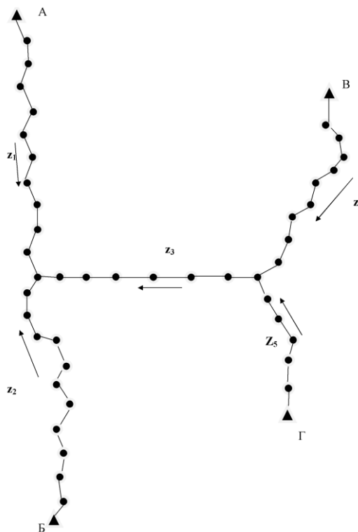
Рис.1 Схема проекта сети полигонометрии
